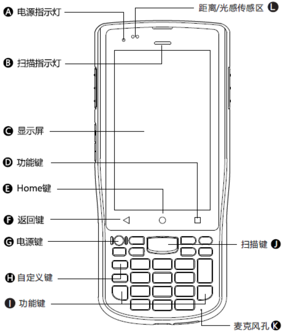
EDA50K-X 无线终端前面板图
