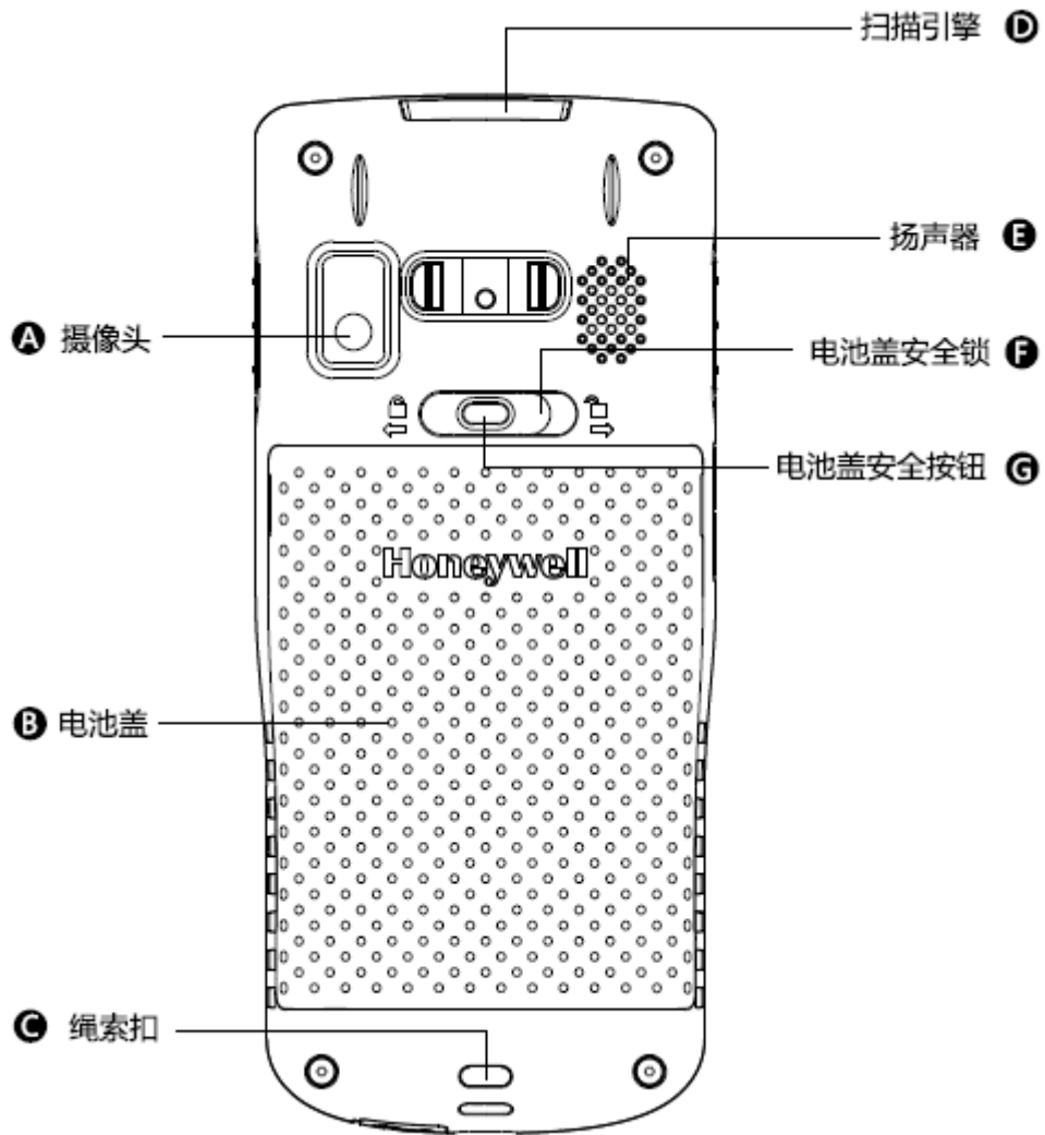
EDA50K-X 无线终端后面板图
