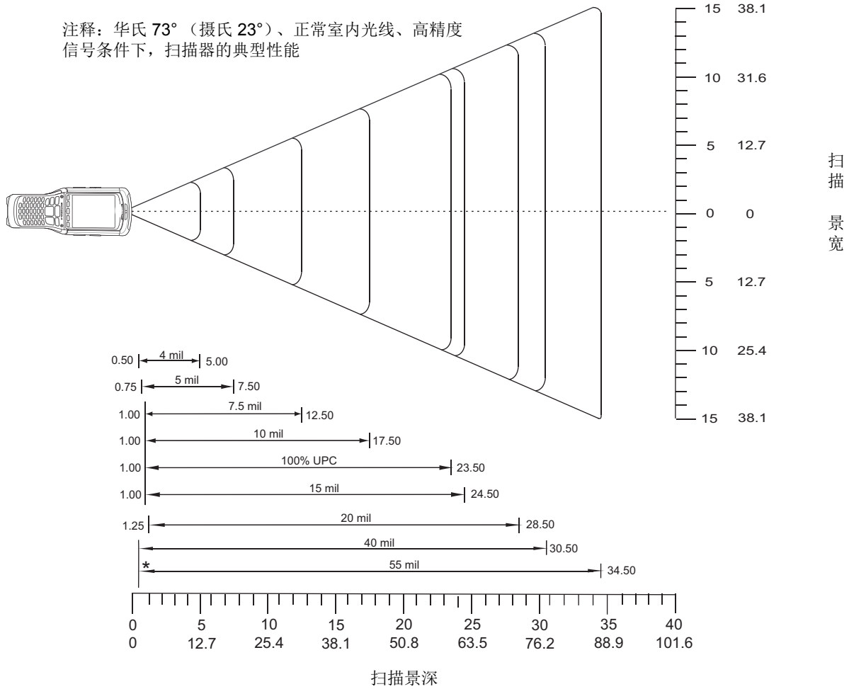
图 4-4 MC9500-K 激光扫描器 47° 解码带
