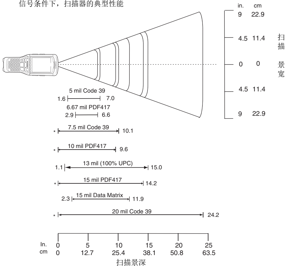
图 4-8 MC9500-K 成像器解码范围
