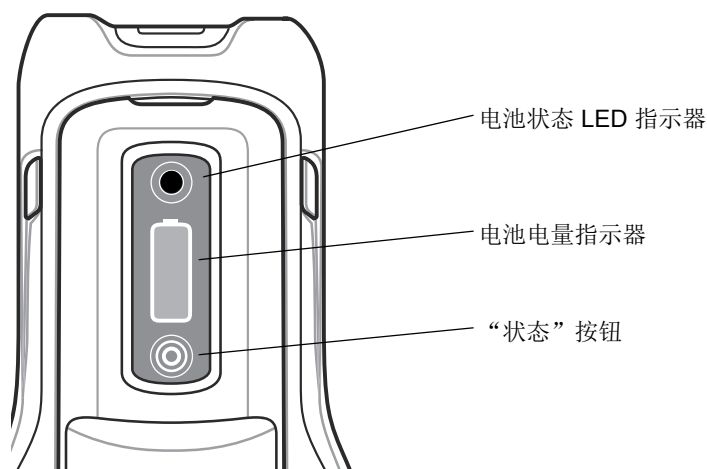
图 2-4 电池装在 MC9500-K 中
