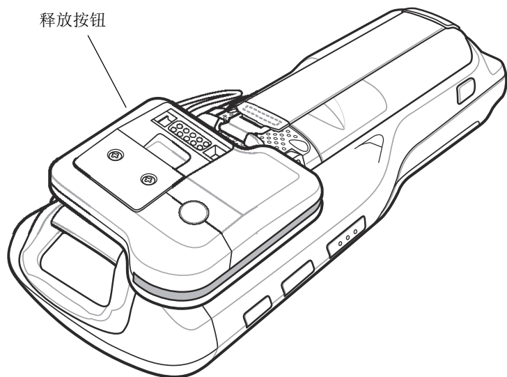
图 8-11 MSR 安装
