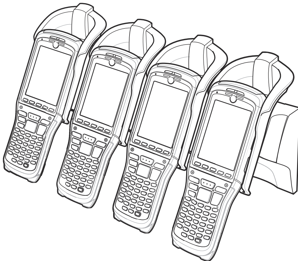
图 8-5 带导杯选件的 MC9500-K 四槽通讯座（仅限于充电）
