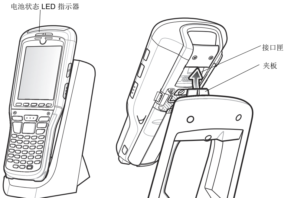
图 8-2 MC9500-K 电池充电
