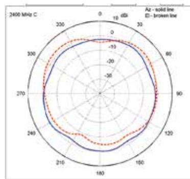
2.4 GHz - 4 dBi 天线
