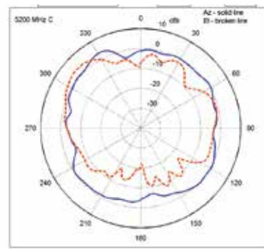
5 GHz - 6 dBi 天线
